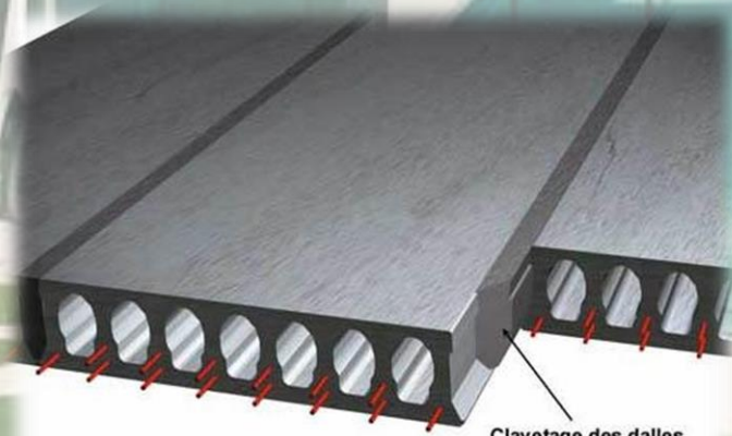
Clavetage des dalles coulé sur chantier
