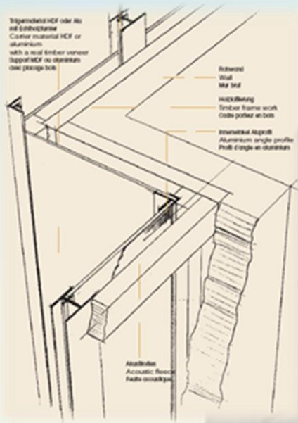
تفصيلية توضح الكسوة الخشبية
