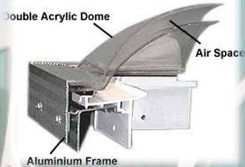
القطاع يوضح الطبقة العازلة في القبة
