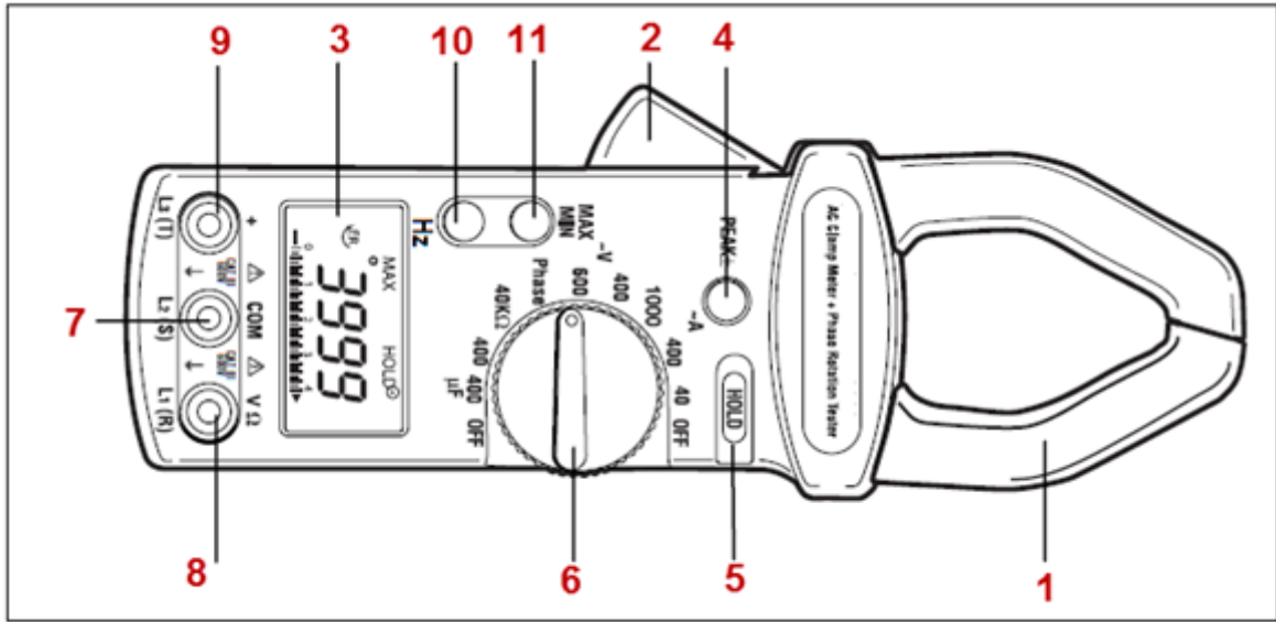
الشكل رقم (١٧) : أحد أنواع الكلامبيتر موضحاً به أجزأه المختلفة
