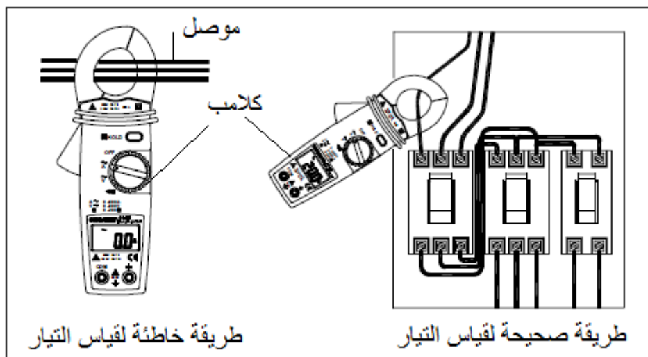
الشكل رقم (١٩): الطريقة الصحيحة لقياس التيار في الموصل
