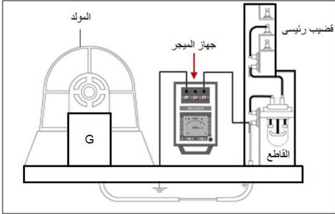
الشكل رقم ( ١٢ ) : قياس مقاومة العزل بين ملفات أحد الأوجه والأرضى لمولد التوربينة
