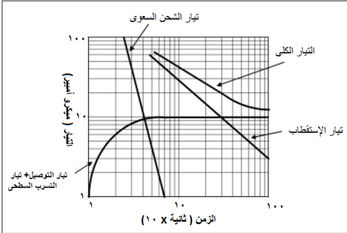
الشكل رقم (٨) : مكونات التيار المار في العزل أثناء قياس المقاومة
