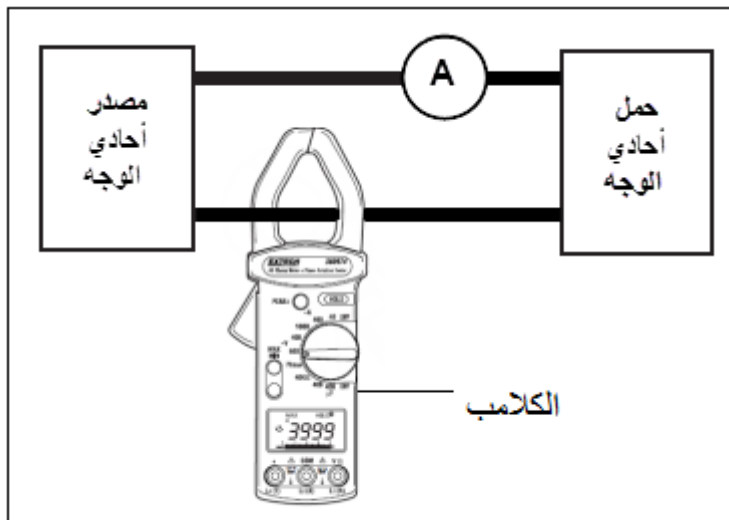
الشكل رقم (٢٦) : قياس التيار باستخدام الكلامبيتر
