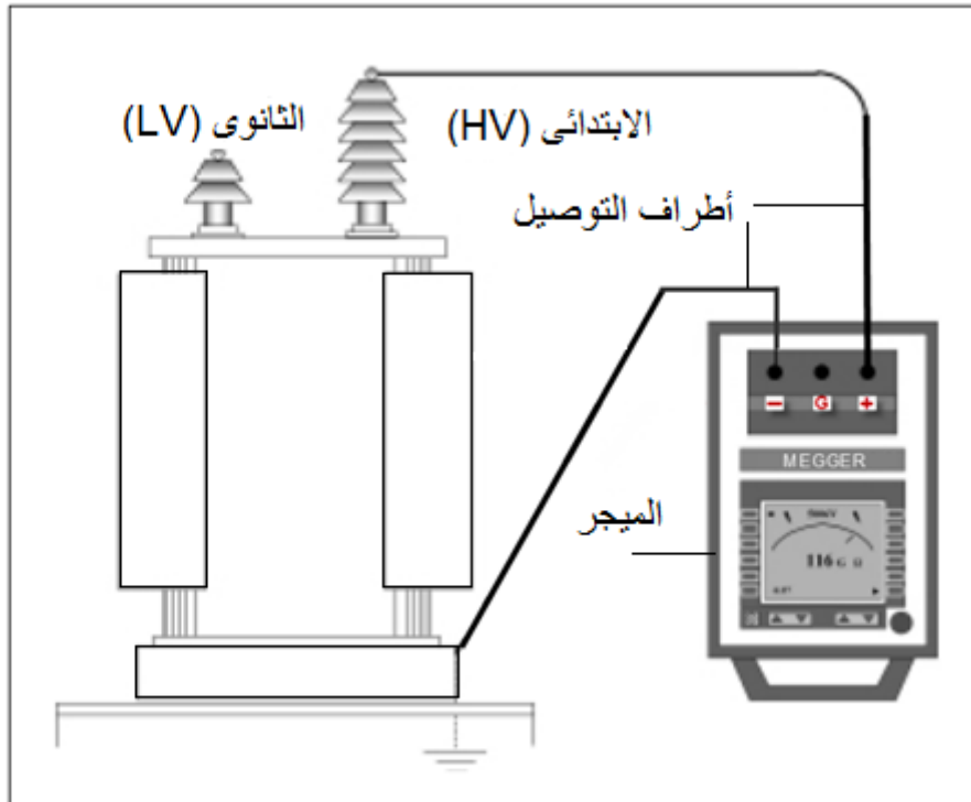
الشكل رقم (١١) : قياس مقاومة العزل بين ملفات الجهد العالي والأرضي لمحور كهربي
