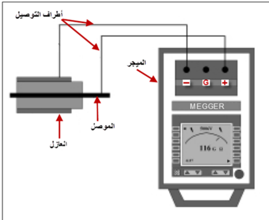
الشكل رقم (٩) : قياس عزل كابل ذو موصل واحد
