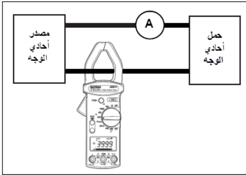
الشكل رقم (٢٠) : قياس التيار باستخدام الكلامبميتر
