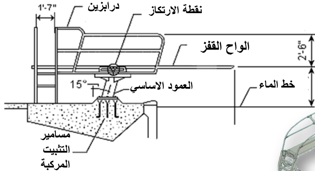
نموذج لألواح الغطس في مستوى سطح الحمام
