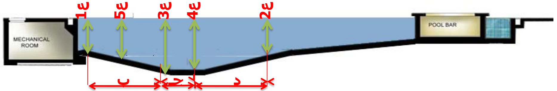
قطاع طولى بالحمام يوضح الميول في الارضية
