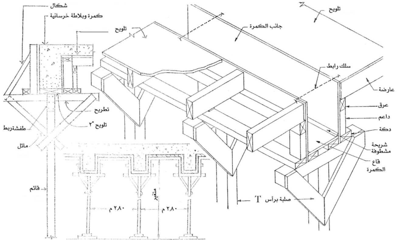
الشكل رقم (٤-٥): الشدات الخشبية للكمرات.
