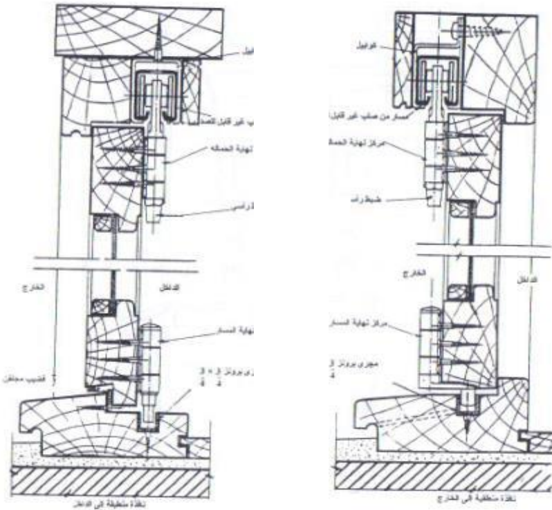
قطاعات راسية
