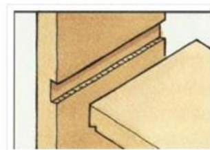
نقر ولسان زاوية
