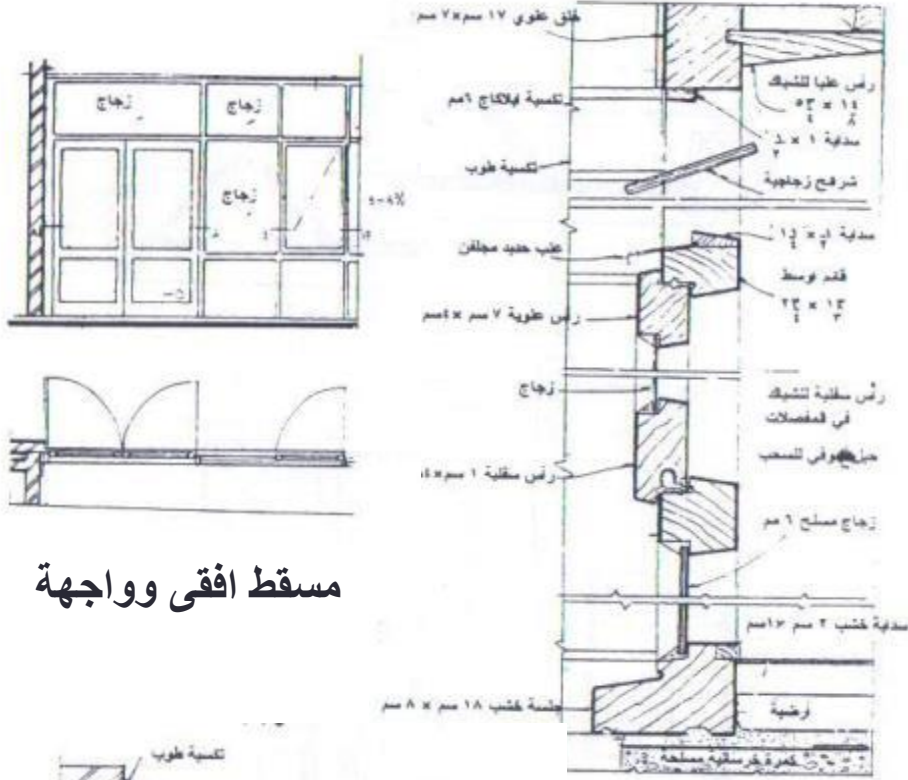
قطاع
