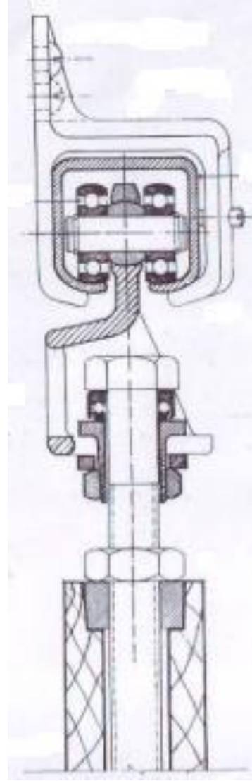
التثبيت جانبي
