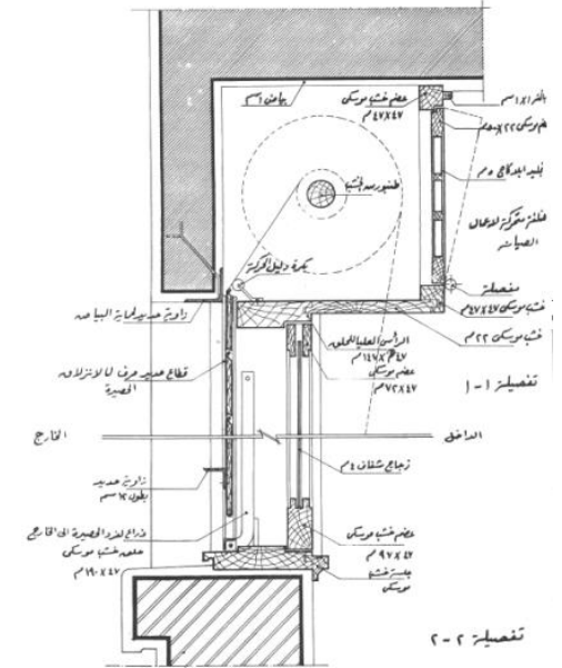
تفصيلات
