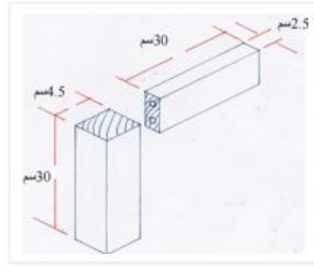
وصلة دسر
