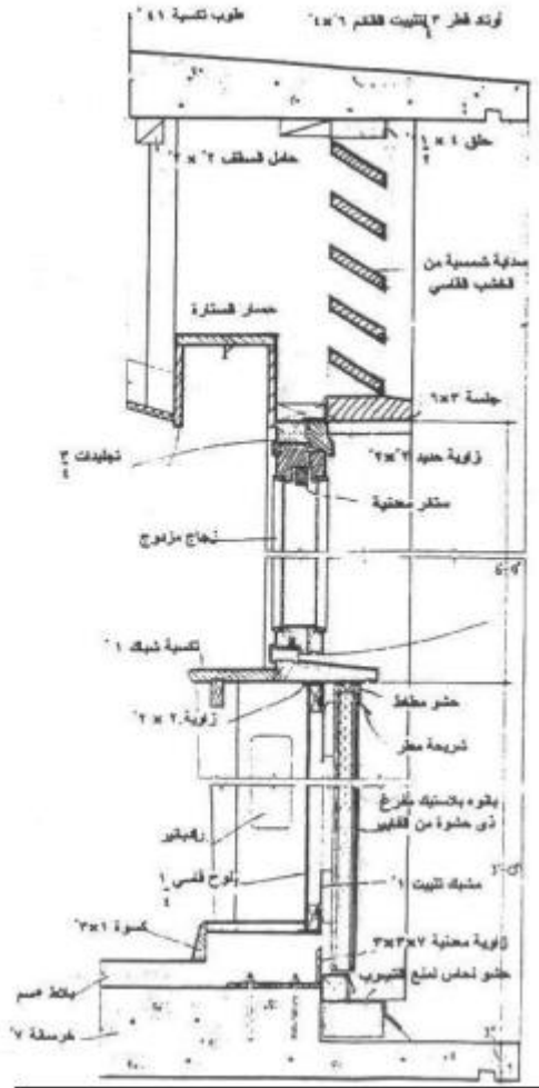
قطاع
