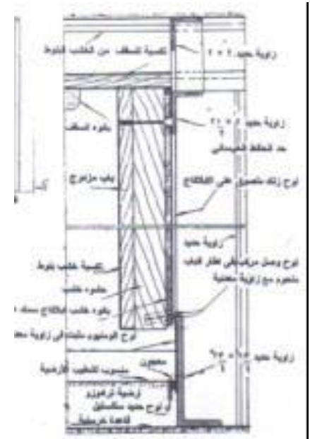
قطاع ا- ا
