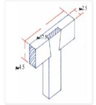
تعشيق ذيل الصمامة T
