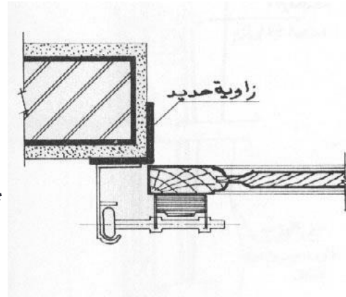
* مسقط أفقي للباب المنزلق لأعلى
