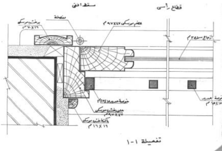
مسقط افقى
