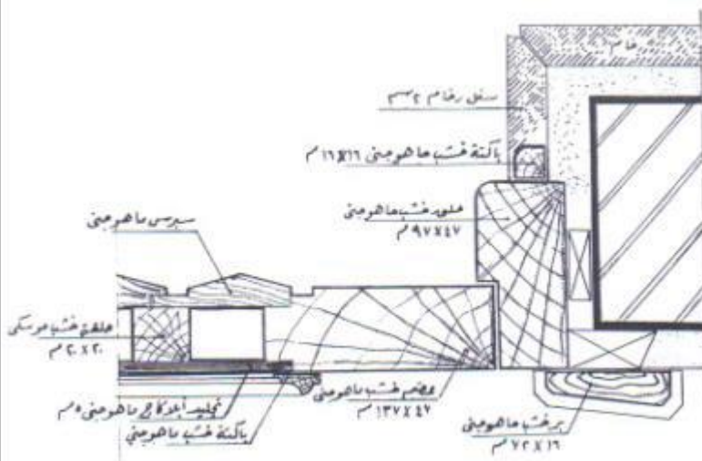
تفصيلة 3 - 3 مسقط افقى
