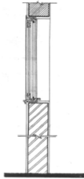
قطاع
